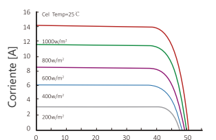
Características del panel a una temperatura constante a 25°C y niveles variables de irradiancia
