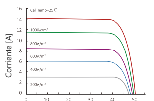
Características del panel a una temperatura constante a 25°C y niveles variables de irradiancia
