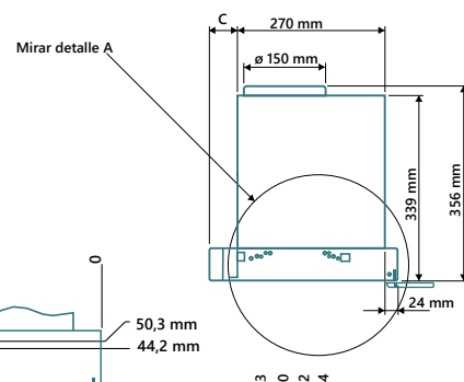
Detalle A Escala 1:4
