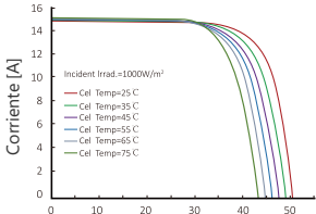
Características del panel a una temperatura variable y niveles de irradiancia 1000W/m²
