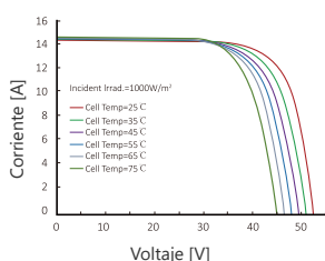
Características del panel a una temperatura variable y niveles de irradiancia 1000W/m 2
